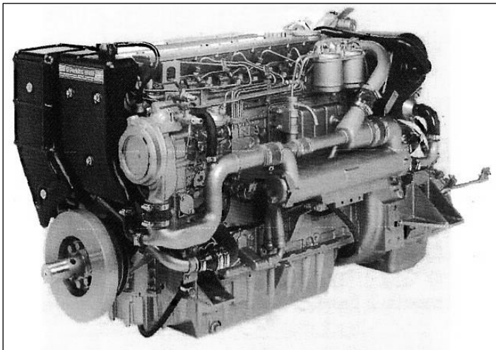
Twee Perkins M215C 158 kW / 215 Pk 4-takt diesel voor de aandrijving van de Stork centrifugaalpompen.
