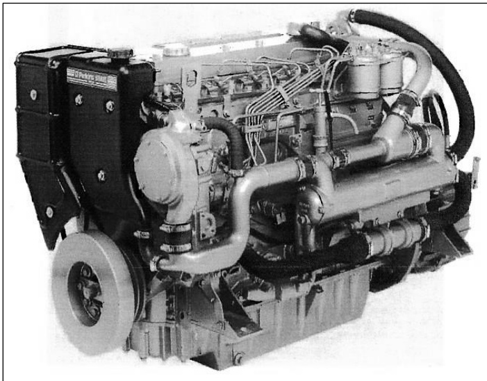
Twee Perkins M130C 99 kW / 135 Pk 4-takt diesel voor de voortstuwing van de blusboot.
